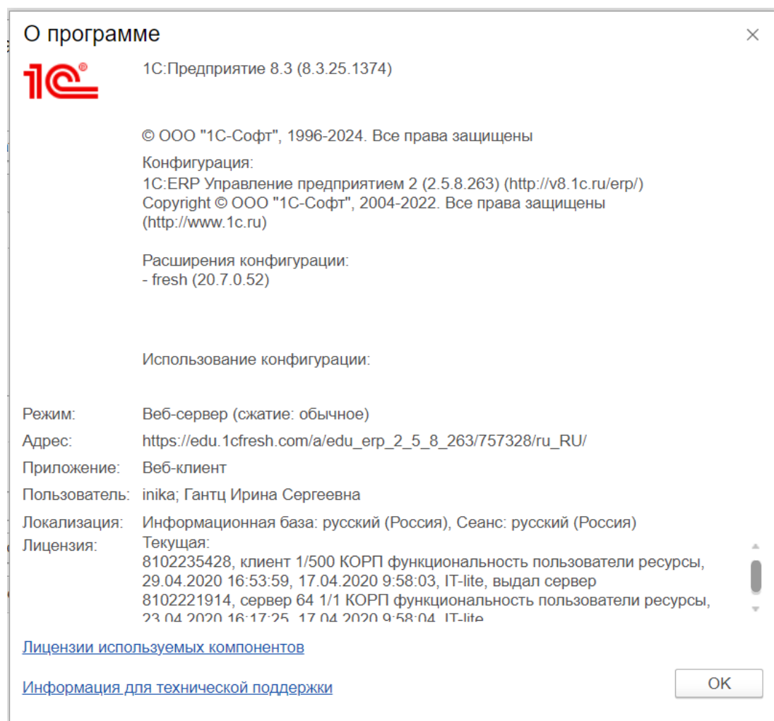
Рисунок 1. О программе
